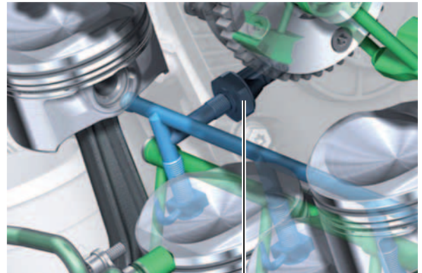
Öldruckschalter Stufe 3 F447 s522_046
