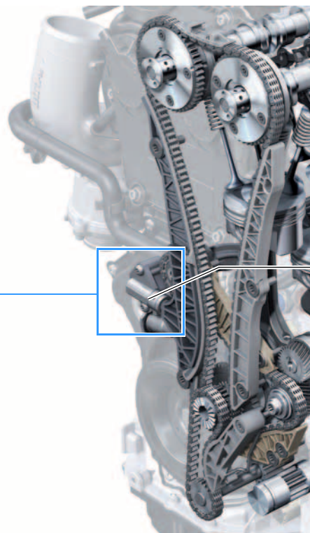
Kettenspanner mit Sichtfenster zur Kettenlängungs-Diagnose
